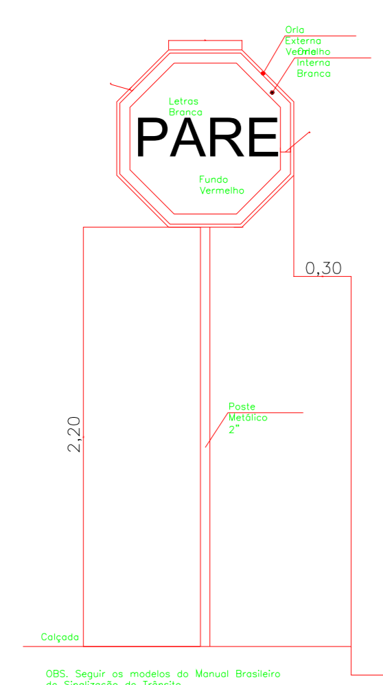
DETALHE PLACA PARE - R-1
