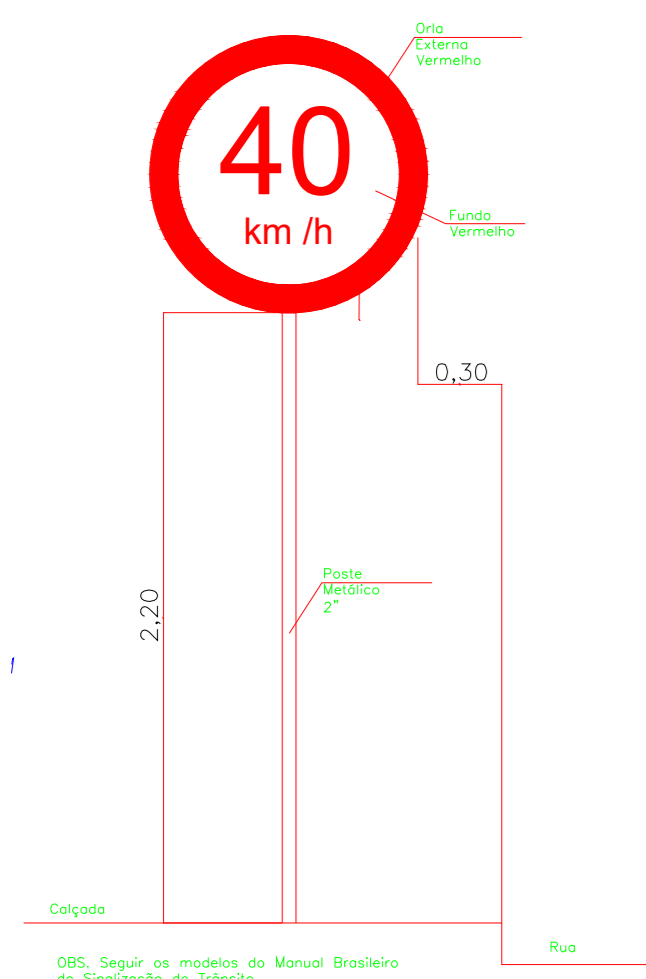
DETALHE PLACA VELOCIDADE MÁXIMA R-19 (40 km/h)
