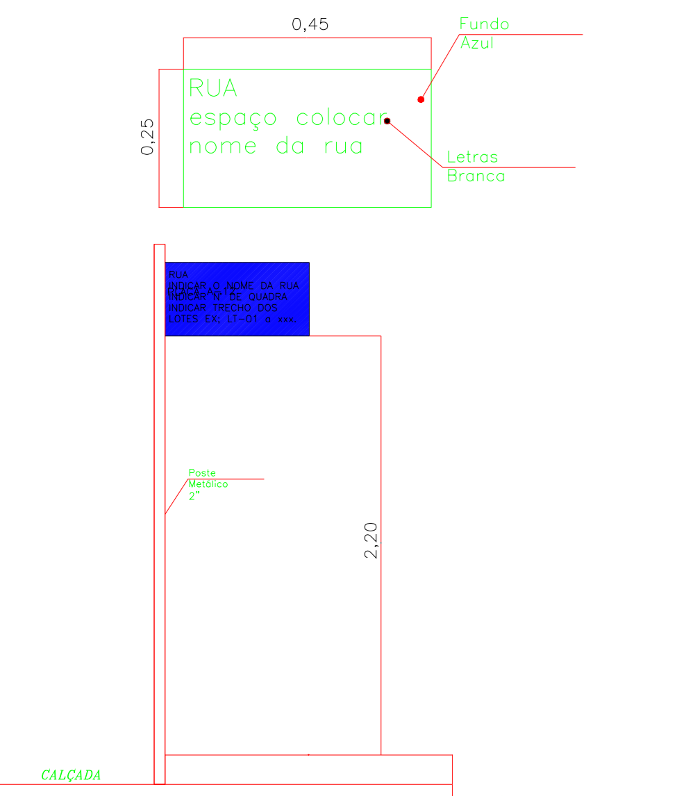
DETALHE PLACA DENOMINATIVAS DE LOGRADOURO PÚBLICOS
