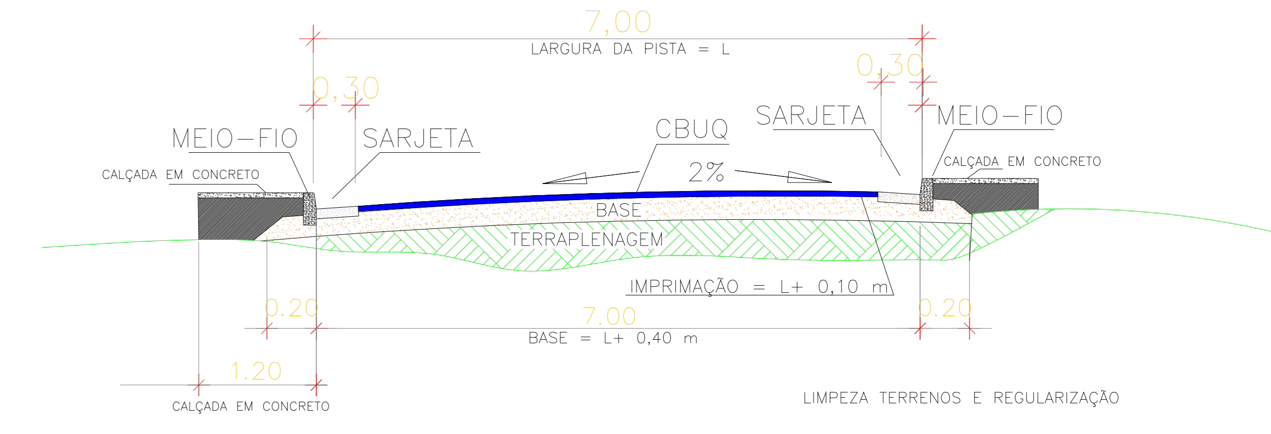
SEÇÃO TIPO DE PAVIMENTAÇÃO e TERRAPLANAGEM Sem escala
