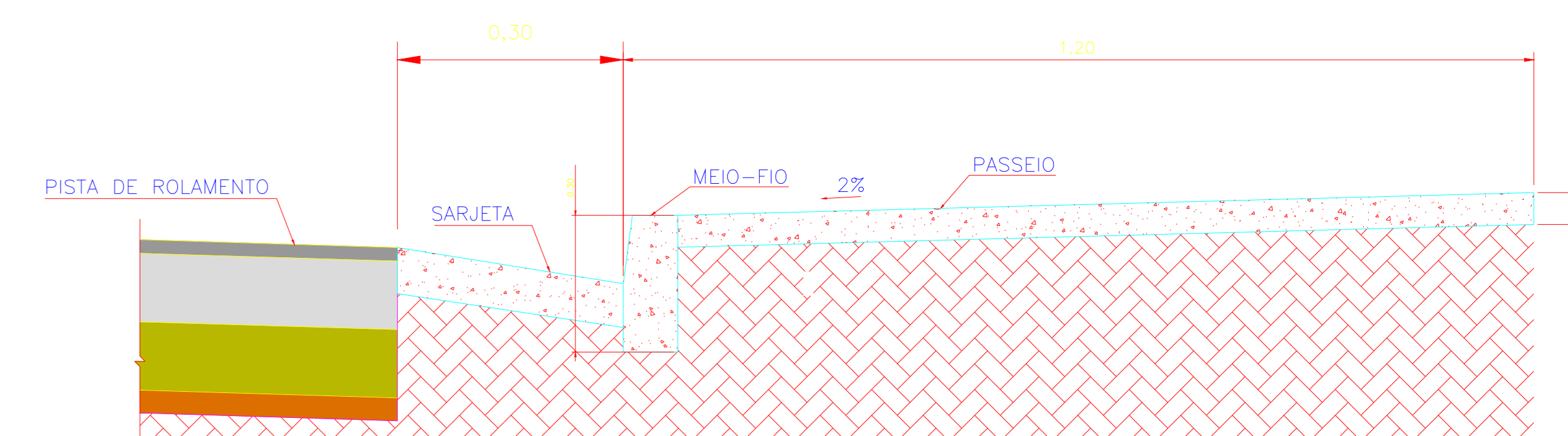
DETALHE DO MEIO-FIO E SARJETA ESC. 1:25
