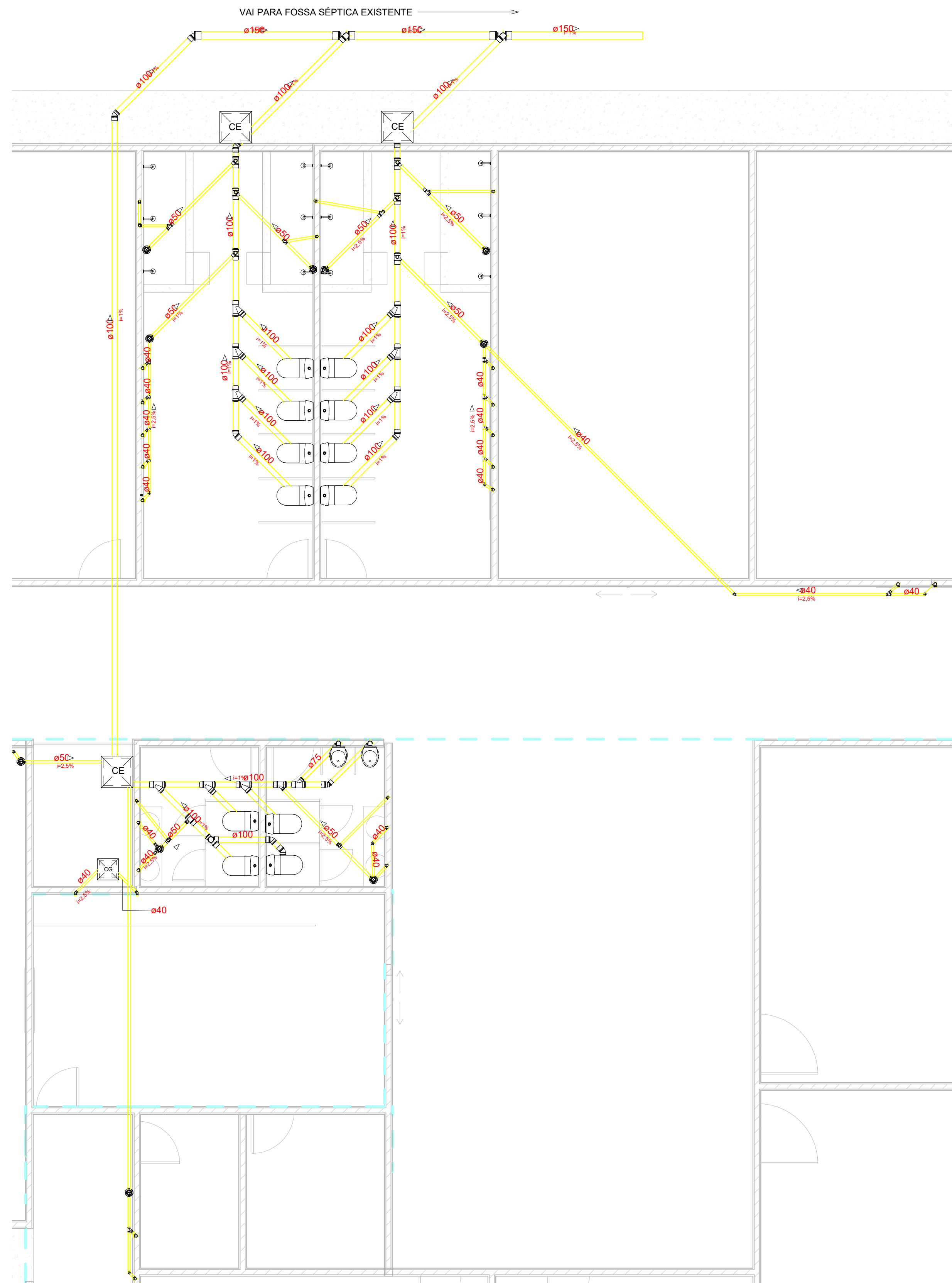
1 PLANTA BAIXA - ESGOTO 1 : 50
